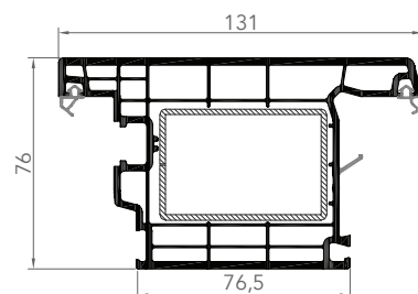
7649E OUVRANT DE PORTE À OUVERTURE VERS L'EXTÉRIEUR
