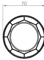
7254 CONNECTEUR TUBULAIRE
