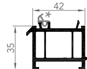
7257 PROFILÉ SOUS-DORMANT
