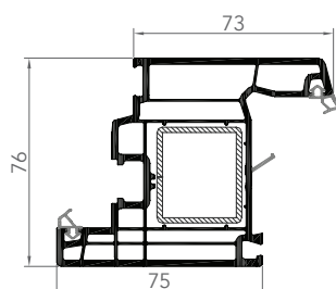
7641AE OUVRANT DE PORTE
