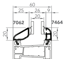
7062-7464 PARCLOSE DOUBLE VITRAGE 20mm
