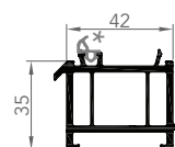
7257 PROFILÉ SOUS-DORMANT
