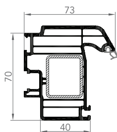
ADAPTATEUR DE PORTE
