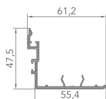
A020559 INTERVERROUILLAGE EN ALUMINIUM POUR OUVRANT 7422
