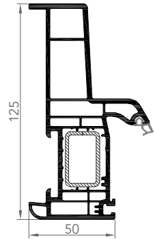
DORMANT MONOBLOC 125
