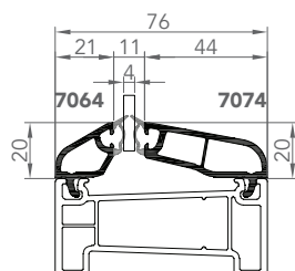
7064-7074 PARCLOSE SIMPLE VITRAGE 4mm
