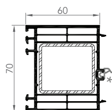
7281 ÉLARGISSEUR 70/60
