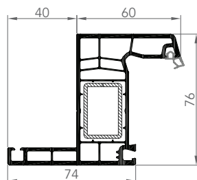
7616AE DORMANT DE RÉNOVATION
