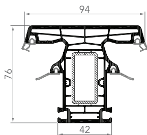
7632E MENEAU
