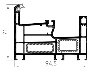
DORMANT FIXE POUR COULISSANT
