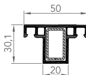
7409 OUVRANT COULISSANT CÔTÉ MENEAU
