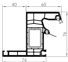
7607E DORMANT DE RÉNOVATION
