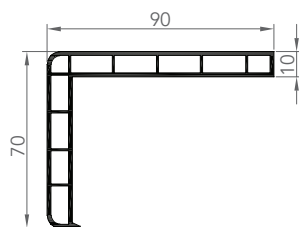
7288 CORNIÈRE D'HABILLAGE
