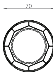
7254 CONNECTEUR TUBULAIRE
