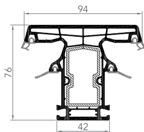
7633E MENEAU
