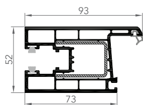
OUVRANT COULISSANT
