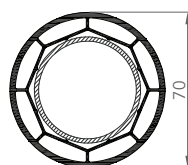
7254 CONNECTEUR TUBULAIRE
