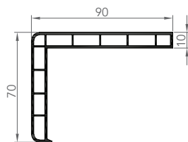
6019 CORNIÈRE D'HABILLAGE
