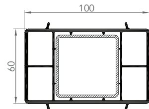
6051 TUBE RECTANGULAIRE 60x100
