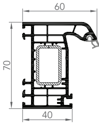
DORMANT
