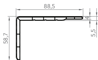
7288 CORNIÈRE D'HABILLAGE
