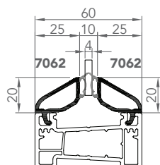
7062-7062 PARCLOSE SIMPLE VITRAGE 4mm
