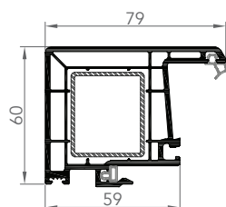
MENEAU D'INTERVERROUILLAGE
