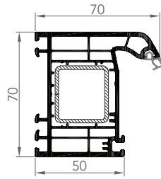
DORMANT
