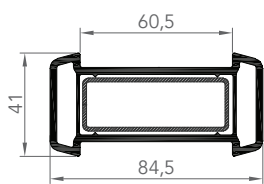
6013 MOUSTIQUAIRE LARGE
