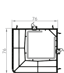
7662 CONNECTEUR D'ANGLE 90°
