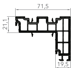
1703 CACHE INTÉRIEUR DE SEUIL HST
