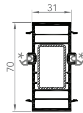
7256 PROFILÉ DE CONNEXION
