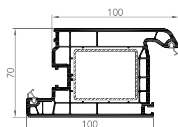
OUVRANT DE PORTE
