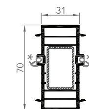
7256 PROFILÉ DE CONNEXION
