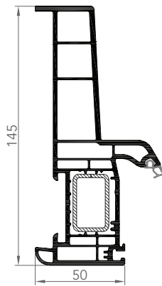
DORMANT MONOBLOC 145
