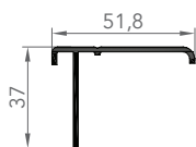
6021 HABILLAGE
