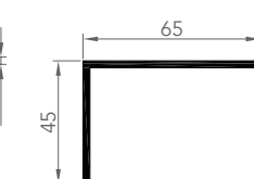
6056 CORNIÈRE D'HABILLA
