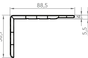
7288 CORNIÈRE D'HABILLAGE
