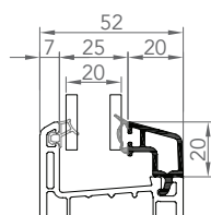
6307 PARCLOSE DOUBLE VITRAGE 20mm
