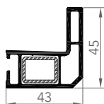
7407 RAIL DE COULISSEMENT DU CADRE DE MOUSTIQUAIRE
