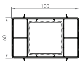
6051 TUBE RECTANGULAIRE 60x100
