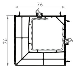
7662 CONNECTEUR D'ANGLE 90°
