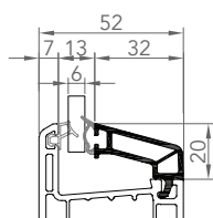
6308 PARCLOSE SIMPLE VITRAGE 6-7 mm
