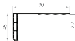
6055 CORNIÈRE D'HABILLAGE
