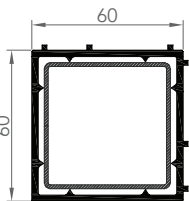
6020 TUBE CARRÉ 60x60
