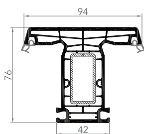
7638E MENEAU
