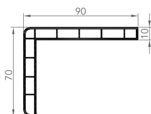
6019 CORNIÈRE D'HABILLAGE
