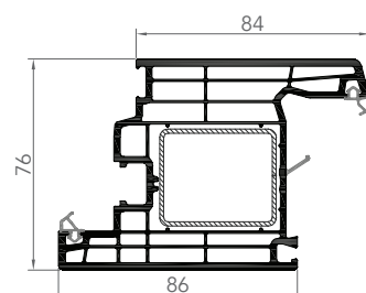
7644E OUVRANT DE PORTE
