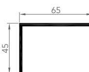
6056 CORNIÈRE D'HABILLAGE
