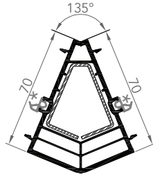
7253 CONNECTEUR D'ANGLE 135°
