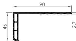
6055 CORNIÈRE D'HABILLAGE
