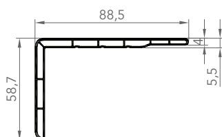
7288 CORNIÈRE D'HABILLAGE
