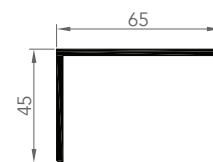
6056 CORNIÈRE D'HABILLAGE
