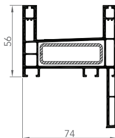
DORMANT COULISSANT DE RÉNOVATION
