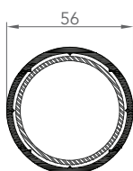
6016 CONNECTEUR TUBULAIRE
