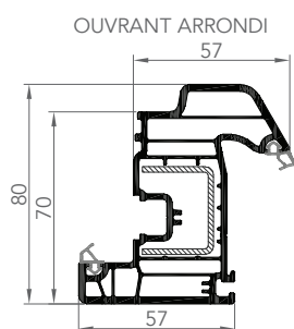
7054 7054E 7054AE
