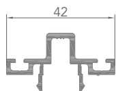
AB01014 PROFIL DE CONNEXION DE L'OUVRANT 6661
