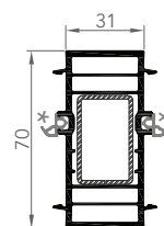
7256 PROFILÉ DE CONNEXION
