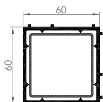
6020 TUBE CARRÉ 60x60
