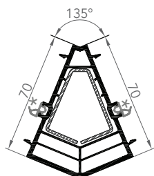
7253 CONNECTEUR D'ANGLE 135°
