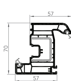
OUVRANT
