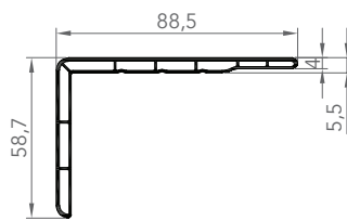
7288 CORNIÈRE D'HABILLAGE
