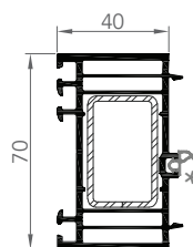
7280 ÉLARGISSEUR 70/40
