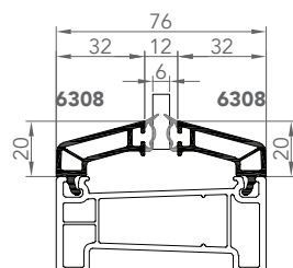
6308-6308 PARCLOSE DOUBLE VITRAGE 6mm
