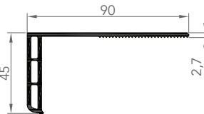
6055 CORNIÈRE D'HABILLAGE
