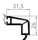
7651 PARCLOSE DOUBLE VITRAGE 24mm
