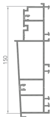
AB02001 SEUIL HAUT EN ALUMINIUM (6695)
