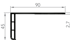
6056 CORNIÈRE D'HABILLAGE
