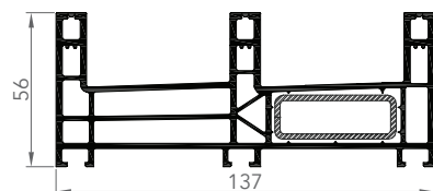
DORMANT COULISSANT À TROIS RAILS
