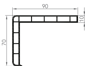
6019 CORNIÈRE D'HABILLAGE
