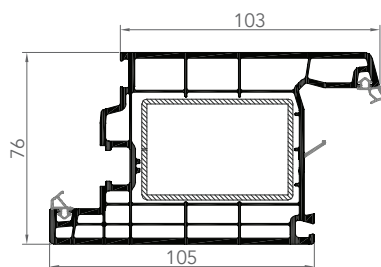
7645AE OUVRANT DE PORTE
