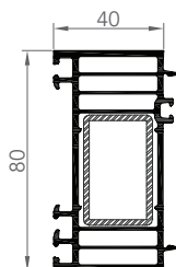
7282 ÉLARGISSEUR 80/40
