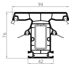
7631AE MENEAU
