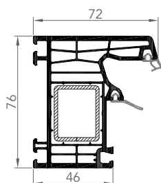
7602E DORMANT
