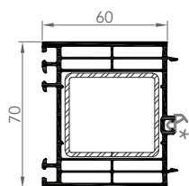
7281 ÉLARGISSEUR 70/60
