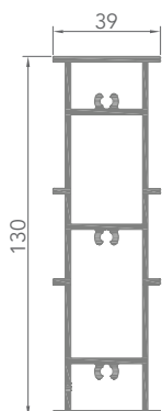
AB02005 RENFORT EN ALUMINIUM DU DORMANT (6767)
