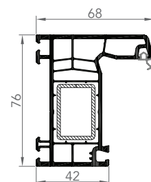
7611E DORMANT
