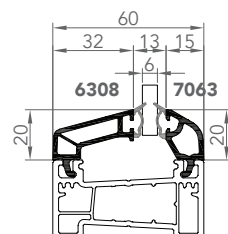
6308-7063 PARCLOSE DOUBLE VITRAGE 6mm
