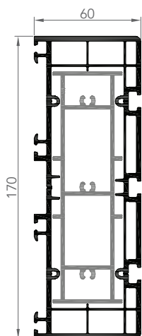
1701 DORMANT COULISSANT À LEVAGE
