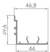
A020560 INTERVERROUILLAGE EN ALUMINIUM DE L'OUVRANT COULISSANT
