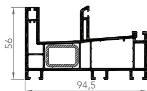
DORMANT FIXE POUR COULISSANT
