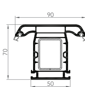
MENEAU
