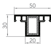
7409 OUVRANT COULISSANT CÔTÉ MENEAU
