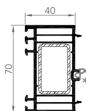
7280 ÉLARGISSEUR 70/40
