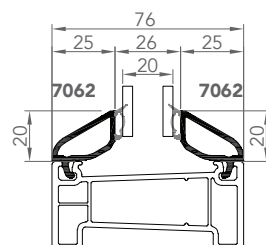
7062-7062 PARCLOSE DOUBLE VITRAGE 20mm
