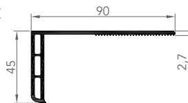
6055 CORNIÈRE D'HABILLAGE
