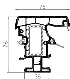
7640E MENEAU MOBILE
