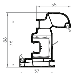
7626AE OUVRANT ARRONDI
