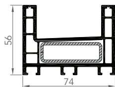
DORMANT COULISSANT
