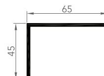
6056 CORNIÈRE D'HABILLAGE
