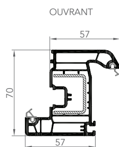
7053 7053E 7053AE
