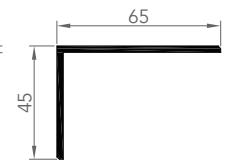
6056 CORNIÈRE D'HABI
