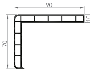
6019 CORNIÈRE D'HABILLAGE
