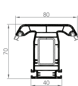
MENEAU
