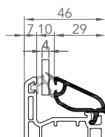
7088 PARCLOSE DOUBLE VITRAGE 4mm
