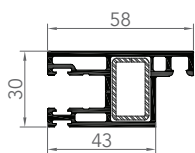
7408 OUVRANT COULISSANT DE MOUSTIQUAIRE
