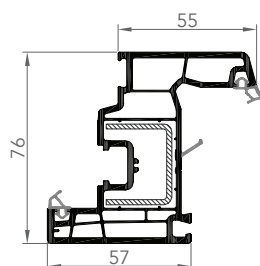
7621AE OUVRANT
