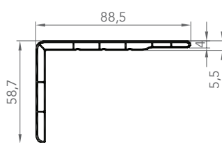
7288 CORNIÈRE D'HABILLAGE
