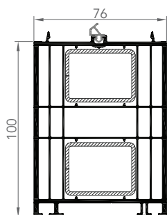
7663 ÉLARGISSEUR 76/100
