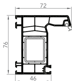
7612AE DORMANT
