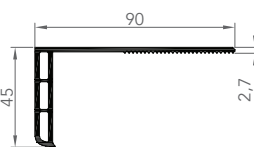
6055 CORNIÈRE D'HABILLAGE
