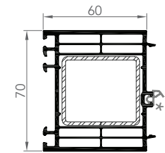
7281 ÉLARGISSEUR 70/60
