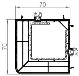
7252 CONNECTEUR D'ANGLE 90°
