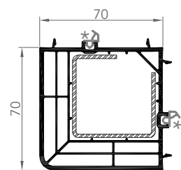
7252 CONNECTEUR D'ANGLE 90°
