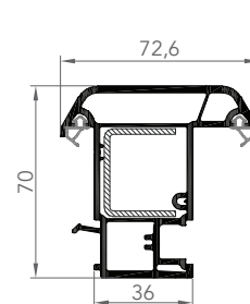
MENEAU MOBILE
