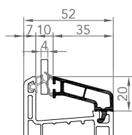
6306 PARCLOSE SIMPLE VITRAGE 4mm
