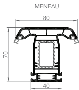
7056 7056E 7056AE
