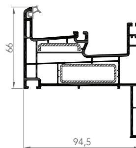
DORMANT FIXE DE RÉNOVATION POUR COULISSANT
