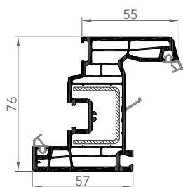
7622E OUVRANT
