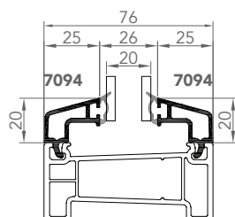
7094-7094 PARCLOSE DOUBLE VITRAGE 20mm
