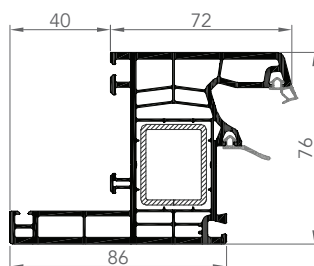
7608E DORMANT DE RÉNOVATION
