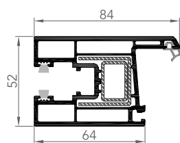
OUVRANT COULISSANT
