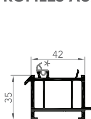
7257 PROFILÉ SOUS-DORMANT
