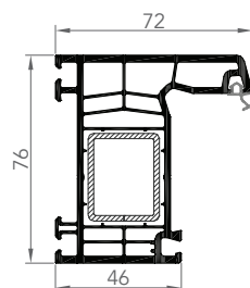
7613E DORMANT
