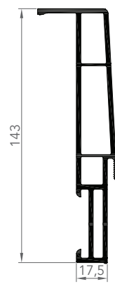
PIÈCE D'APPUI 143
