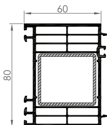
7283 ÉLARGISSEUR 80/60
