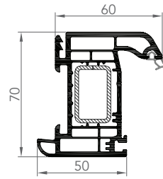
DORMANT
