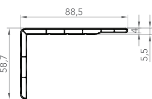
6055 CORNIÈRE D'HABILLAGE
