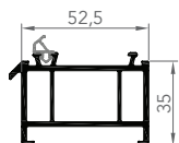
7666 PROFILÉ SOUS-DORMANT
