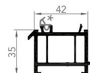
7257 PROFILÉ SOUS-DORM
