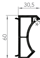
6015 CONNECTEUR D'ANGLE
