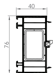
7665 ÉLARGISSEUR 76/40
