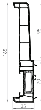
PIÈCE D'APPUI 165
