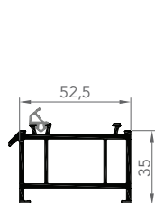
7666 PROFILÉ SOUS-DORMANT
