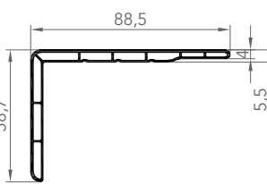
7288 CORNIÈRE D'HABILLAGE
