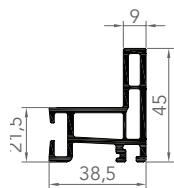
7465 RAIL COULISSANT DU CADRE DE MOUSTIQUAIRE
