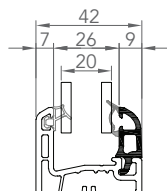
7464 PARCLOSE DOUBLE VITRAGE 20mm
