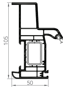
DORMANT MONOBLOC 105
