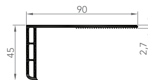
6055 CORNIÈRE D'HABILLAGE
