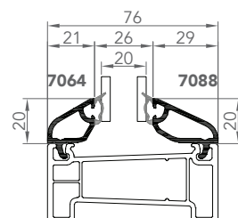
7064-7088 PARCLOSE DOUBLE VITRAGE 20mm
