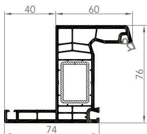
7617E DORMANT DE RÉNOVATION
