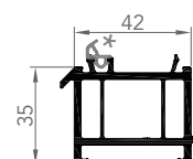
7257 PROFILÉ SOUS-DORMANT
