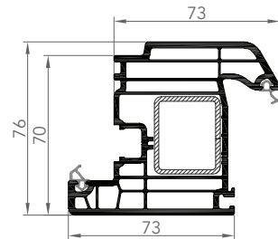
OUVRANT DE PORTE
