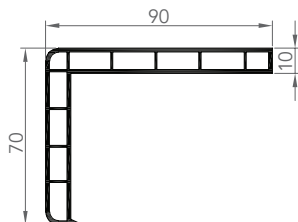
6019 CORNIÈRE D'HABILLAGE
