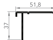
6021 HABILLAGE
