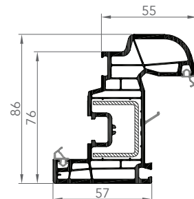
7627E OUVRANT ARRONDI
