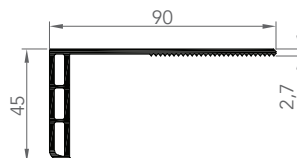
6055 CORNIÈRE D'HABILLAGE
