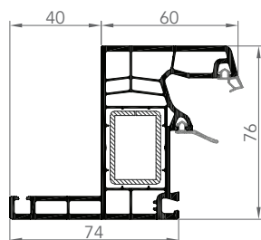
7606AE DORMANT DE RÉNOVATION
