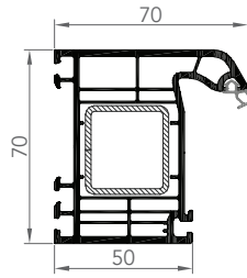
DORMANT
