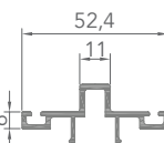
A001961 PROFILÉ DE CONNEXION
