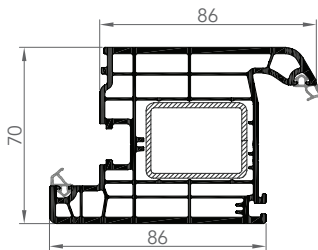
7057 7057E 7057AE
