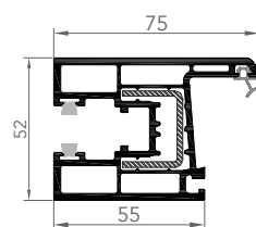
OUVRANT COULISSANT
