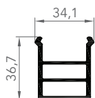
6053 PROFILÉ SOUS-DORMANT
