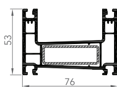
DORMANT COULISSANT
