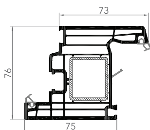
7642E OUVRANT DE PORTE
