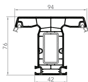
7637AE MENEAU
