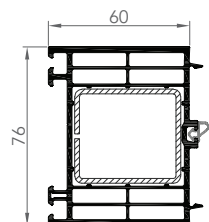
7667 ÉLARGISSEUR 76/60
