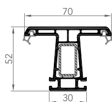
MENEAU COULISSANT
