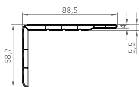
7288 CORNIÈRE D'HABILLAGE
