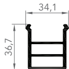
6053 PROFILÉ SOUS-DORMANT
