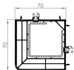
7252 CONNECTEUR D'ANGLE 90°
