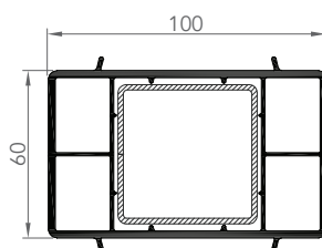
6051 TUBE RECTANGULAIRE 60x100
