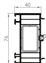
7665 ÉLARGISSEUR 7
