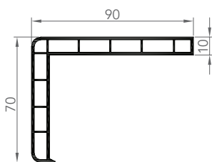
6019 CORNIÈRE D'HABILLAGE
