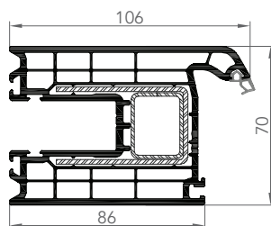
1702 OUVRANT COULISSANT À LEVAGE
