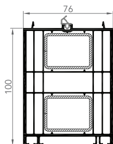
7663 ÉLARGISSEUR 76/100
