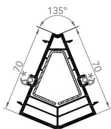
7253 CONNECTEUR D'ANGLE 135°
