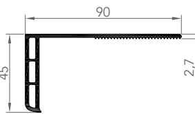
6055 CORNIÈRE D'HABILLAGE
