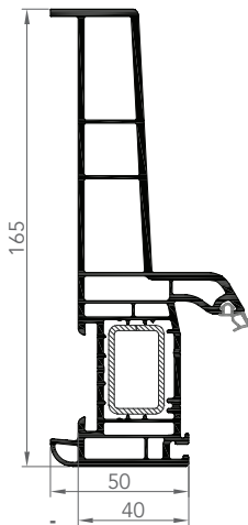
DORMANT MONOBLOC 165
