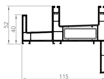
DORMANT COULISSANT DE RÉNOVATION AVEC MOUSTIQUAIRE
