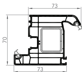
OUVRANT DE PORTE
