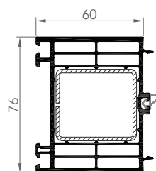
7667 ÉLARGISSEUR 76/60
