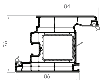
7643AE OUVRANT DE PORTE
