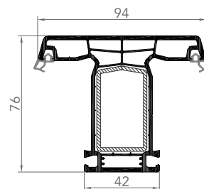
7636AE MENEAU
