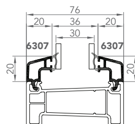
6307-6307 PARCLOSE DOUBLE VITRAGE 30mm
