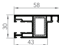
7408 PROFIL D'OUVRANT COULISSANT DE MOUSTIQUAIRE
