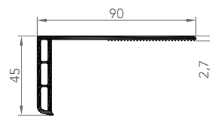
6055 CORNIÈRE D'HABILLAGE
