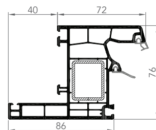
7609AE DORMANT DE RÉNOVATION
