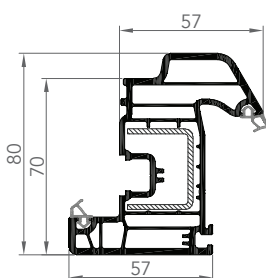
OUVRANT ARRONDI
