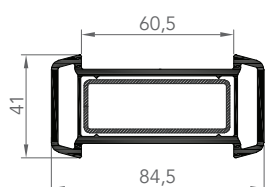
6013 MOUSTIQUAIRE LARGE
