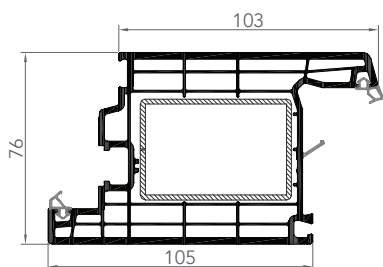
7646E OUVRANT DE PORTE
