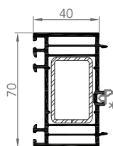
7280 ÉLARGISSEUR 70/40
