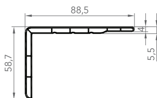
7288 CORNIÈRE D'HABILLAGE
