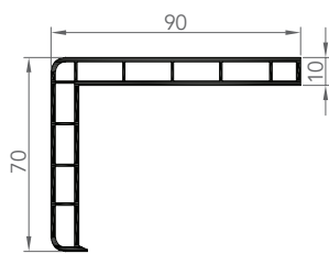
6019 CORNIÈRE D'HABILLAGE
