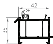
7257 PROFILÉ SOUS-DORMANT
