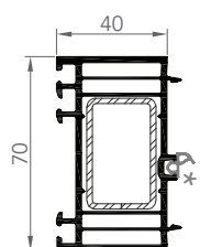
7280 ÉLARGISSEUR 70/40
