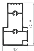
A017581 EXTENSION DE MENEAU
