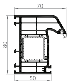
DORMANT
