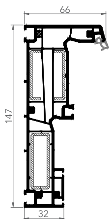
1471E FRAME
