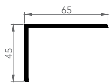
6056 MASKING
