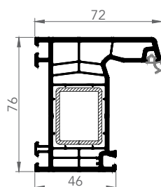
7613E FRAME
