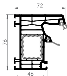
7602E FRAME
