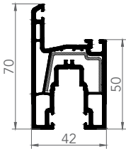
7461E 7461AE
