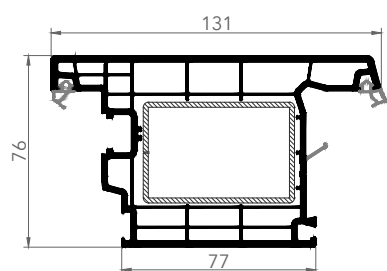
7649E OUTWARD OPENING DOOR SASH
