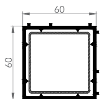
6020 KUTU PROFİLİ
