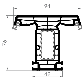
7638E MULLION
