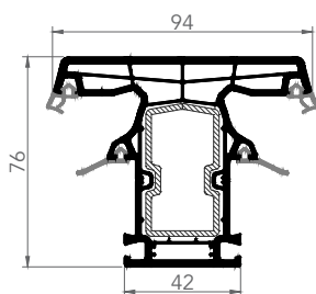
7633E MULLION
