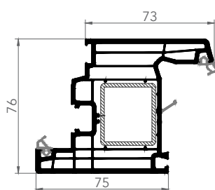
7642E DOOR SASH
