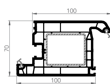
DOOR SASH
