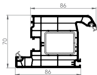
DOOR SASH
