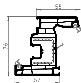
7622E SASH
