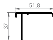
6021 MASKING
