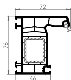
7612AE FRAME
