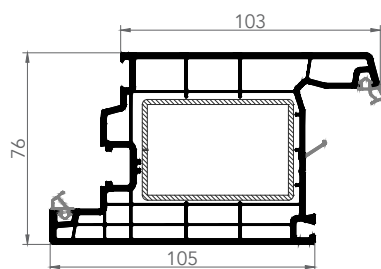
7645AE DOOR SASH
