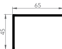
6056 MASKING
