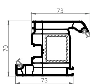
DOOR SASH
