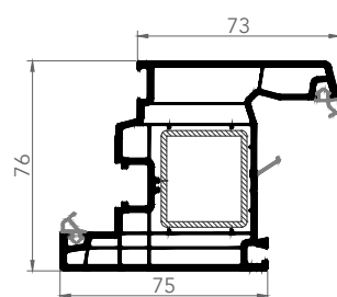
7641AE DOOR SASH
