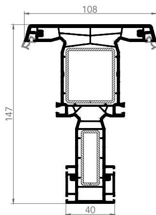
1476E FRAME
