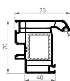
DOOR ADAPTER
