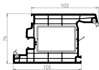
7646E DOOR SASH
