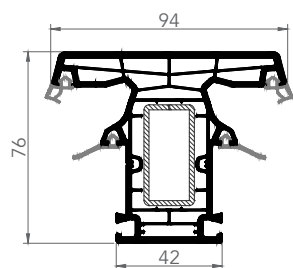
7632E MULLION
