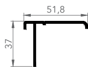
6021 MASKING
