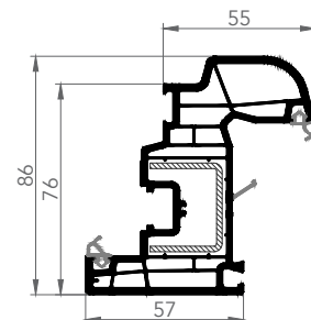
7627E DROPPER SASH
