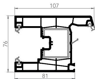
1472E SASH
