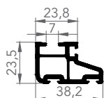
1712 INTERLOCK
