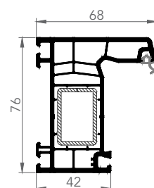
7611E FRAME
