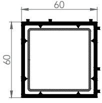
6020 KUTU PROFİLİ
