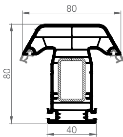
ORTA KAYIT
