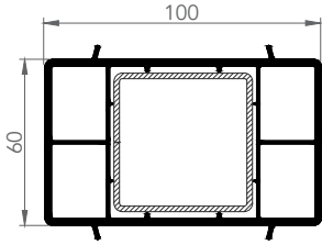
6051 60x100 ODACIKLI KUTU PROFİLİ
