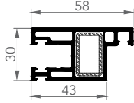
7408 SİNEKLİK KANAT
