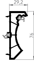
7661 KÖŞE ADAPTÖR
