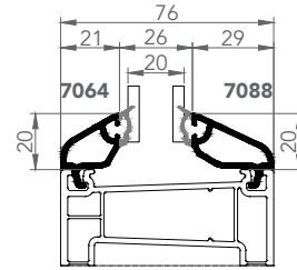
7064-7088 ÇİFT CAM ÇİTASI 20mm
