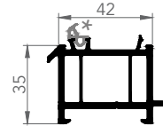
7257 KÖRKASA YÜKSELTME
