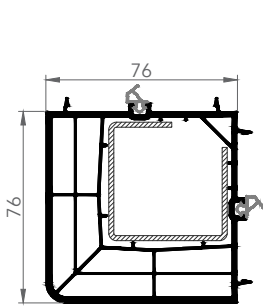
7662 90°KÖŞE ADAPTÖR
