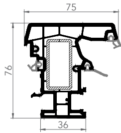
7640E HAREKETLİ ORTAKAYIT
