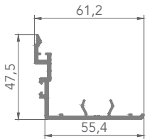
A020559 7422 KANAT İÇİN ALÜMİNYUM INTERLOCK
