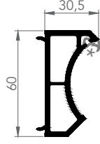
6015 KÖŞE DÖNÜŞ ADAPTÖRÜ
