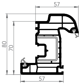
DAMLALIKLI KANAT
