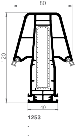
HOLLANDA ORTA KAYIT
