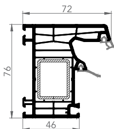
7602E KASA
