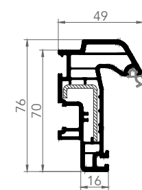
ADAPTÖR KANAT
