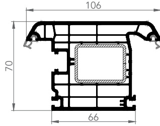
DIŞA AÇILIR KAPI KANAT
