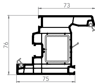
7641AE KAPI KANAT
