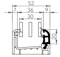
7464 ÜÇLÜ CAM ÇİTASI 30mm
