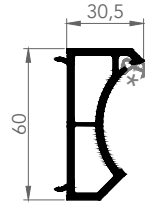
6015 KÖŞE DÖNÜŞ ADAPTÖRÜ
