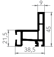
7465 SİNEKLİK RAY KASA
