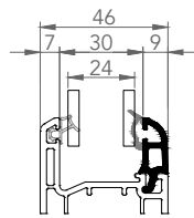
7464 ÜÇLÜ CAM ÇİTASI 24mm
