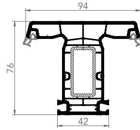
7637AE ORTA KAYIT
