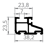
1712 INTERLOK
