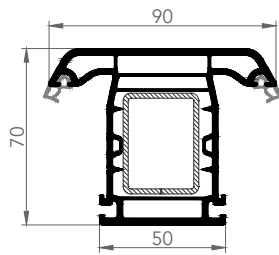
ORTA KAYIT
