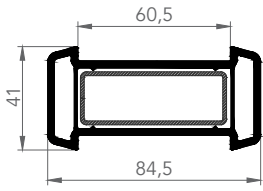
6013 GENİŞ BAĞLANTI
