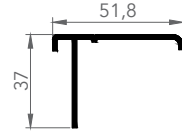
6021 T PERVAZ
