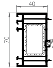
7280 70x40 mm YÜKSELTME
