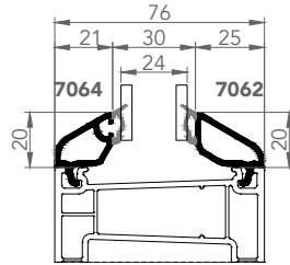
7064-7062 ÇİFT CAM ÇİTASI 24mm
