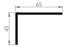
6056 L-PERVAZ
