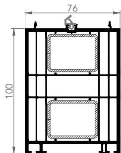
7663 76/100 YÜKSELTME
