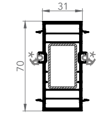
7256 GRİYAJ BAĞLANTISI
