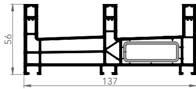
ÜÇ RAYLI SÜRME KASA
