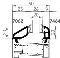
7062-7464 ÇİFT CAM ÇİTASI 20mm
