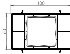
6051 60x100 ODACIKLI KUTU PROFİLİ
