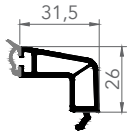
7651 ÇİFT CAM ÇİTASI 24 mm
