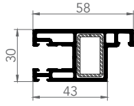
7408 SİNEKLİK KANAT
