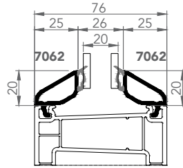
7062-7062 ÇİFT CAM ÇİTASI 20mm
