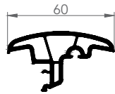
7073 SABİT KANAT DIŞ BİNİ
