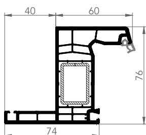
7617E PERVAZLI KASA
