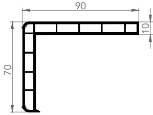
6019 KALIN PERVAZ
