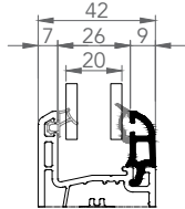
7464 ÇİFT CAM ÇİTASI 20mm
