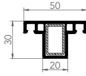
7409 SİNEKLİK KANAT İÇİ ORTAKAYIT
