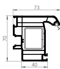
KAPI ADAPTÖR
