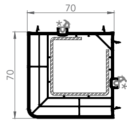
7252 70x70 KUTU "90 DERECE"
