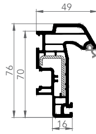
ADAPTÖR KANAT
