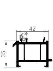
7257 KÖRKASA YÜKSELTME
