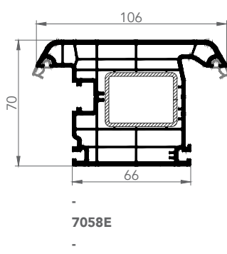
DIŞA AÇILIR KAPI KANAT
