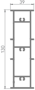
AB02005 ALÜMİNYUM DESTEK PROFİLİ (6767)
