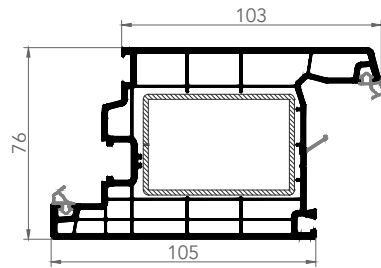
7645AE KAPI KANAT
