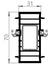
7256 GRİYAJ BAĞLANTISI
