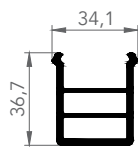
7251 LAMBİRİ PROFİLİ
