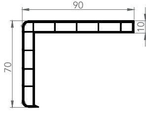
6019 KALIN PERVAZ
