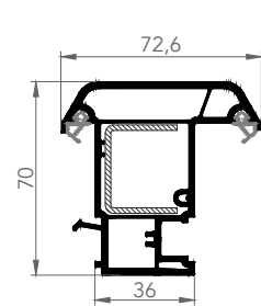
HAREKETLİ ORTA KAYIT
