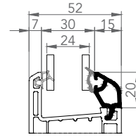
7063 ÇİFT CAM ÇİTASI 24mm
