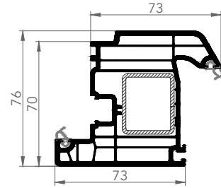
KAPI KANAT
