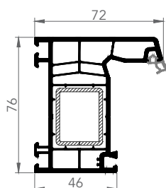
7612AE KASA
