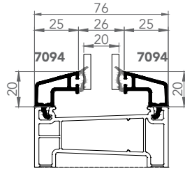
7094-7094 ÇİFT CAM ÇİTASI 20mm
