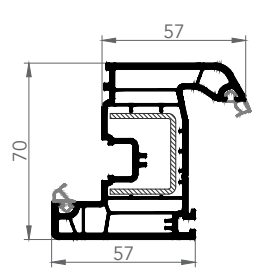
KANAT
