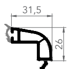
7652 ÇİFT CAM ÇİTASI 24mm
