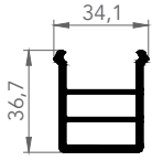
6053 KÖRKASA YÜKSELTME
