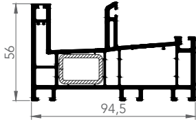
SÜRME SABİT KASA
