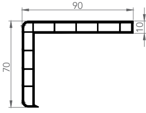
6019 KALIN PERVAZ
