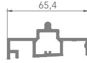
AB02007 ALÜMİNYUM DIŞ EŞİK RAY HAFİF (7430)
