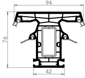
7632E ORTA KAYIT
