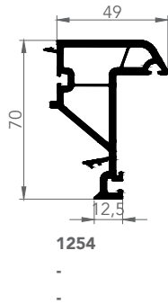
KLİPS PROFİLİ
