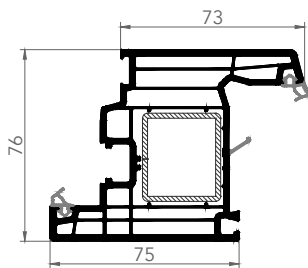
7642E KAPI KANAT
