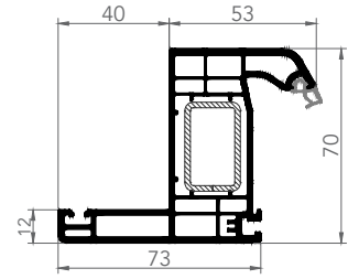
PERVAZLI KASA
