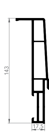
DENİZLİK FRANSA
