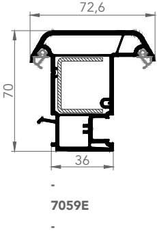
HAREKETLİ ORTA KAYIT
