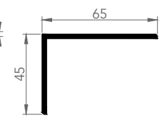
6056 L-PERSİYAN
