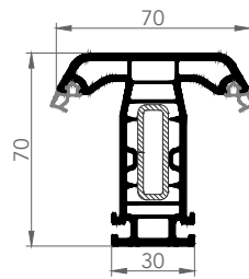
ORTA KAYIT
