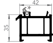
7257 KÖRKASA YÜKSELTME
