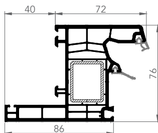
7608E PERVAZLI KASA
