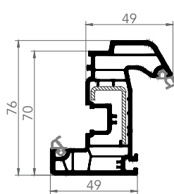
DAMLALIKLI KANAT
