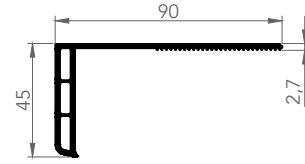
6055 İNCE TIRTIKLI PERVAZ
