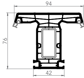
7638E ORTA KAYIT
