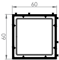
6020 KUTU PROFİLİ
