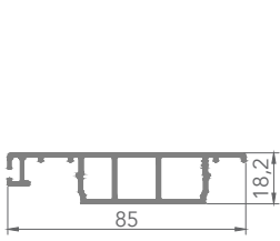
A017270 SÜRME KANAT DİKEY STATİK KAPAMA
