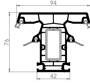
7631AE ORTA KAYIT
