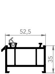
7666 KÖR KASA YÜKSELTME
