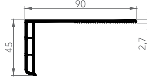
6055 İNCE TIRTIKLı PERVAZ
