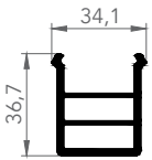
6053 KÖRKASA YÜKSELTME
