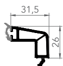
7651 ÇİFT CAM ÇİTASI 24mm
