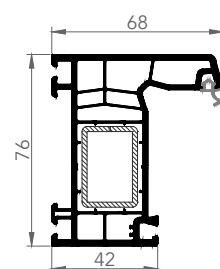
7611E KASA
