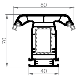
ORTA KAYIT
