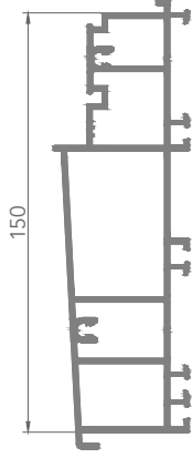
AB02001 ALÜMİNYUM EŞİK YÜKSEK (6695)
