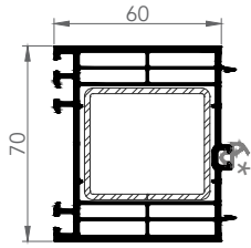
7281 70x60 mm YÜKSELTME
