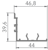
A020560 7461 SÜRME KANAT ALÜMİNYUM INTERLOCK
