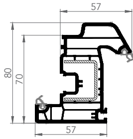
DAMLALIKLI KANAT
