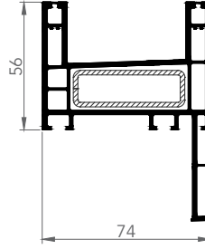
SÜRME PERVAZLI KASA
