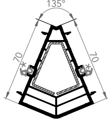
7253 KÖŞE DÖNÜŞ "135 DERECE"
