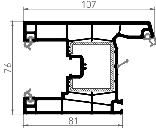
1472E KANAT
