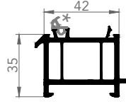
7257 KÖRKASA YÜKSELTME
