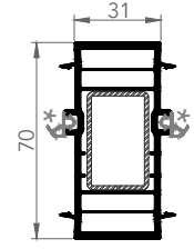
7256 GRİYAJ BAĞLANTISI
