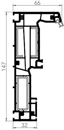
1471E KASA
