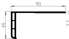
6055 İNCE TIRTIKLİ PERVAZ
