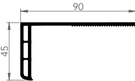
6055 İNCE TIRTIKLı PERVAZ
