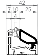
7062 TEK CAM ÇİTASI 4mm
