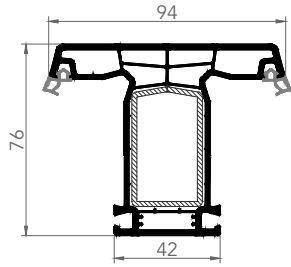
7636AE ORTA KAYIT
