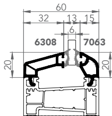
6308-7063 ÇİFT CAM ÇİTASI 6mm
