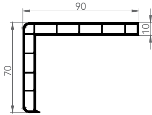
6019 KALIN PERVAZ
