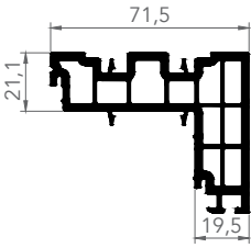
1703 iç EŞİK KAPAMA
