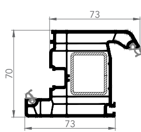
KAPI KANAT
