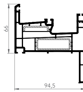
SÜRME SABİT PERVAZLI KASA
