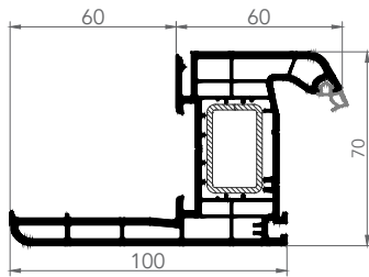
PERVAZLI KASA
