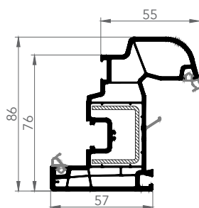
7626AE DAMLALIKLI KANAT
