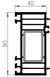
7282 80x40 mm YÜKSELTME
