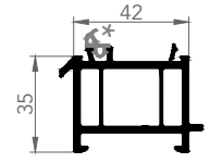
7257 KÖRKASA YÜKSELTME
