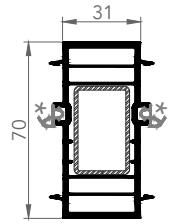
7256 GRİYAJ BAĞLANTISI
