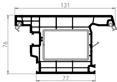
7649E DIŞA AÇILIR KAPI KANAT
