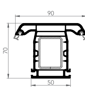
ORTA KAYIT
