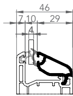
7088 ÇİFT CAM ÇİTASI 4mm
