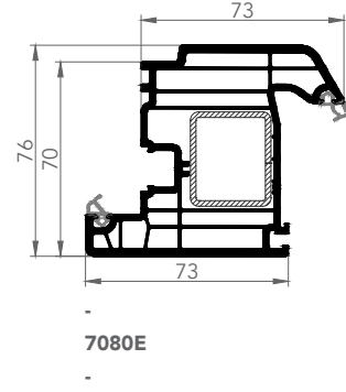
KAPI KANAT
