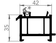
7257 KÖRKASA YÜKSELTME
