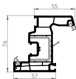
7621AE KANAT
