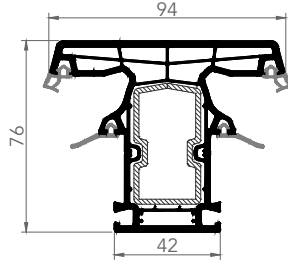
7633E ORTA KAYIT
