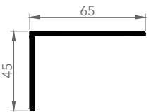
6056 L-PERVAZ
