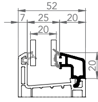
6307 ÇİFT CAM ÇİTASI 20mm
