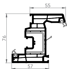
7622E KANAT
