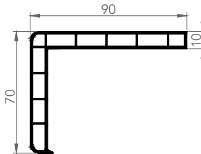
6019 KALIN PERVAZ
