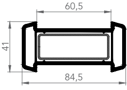
6013 GENİŞ BAĞLANTI
