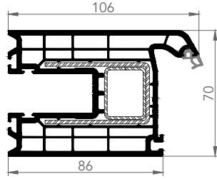
1702 HEBE-SCHIEBE KANAT
