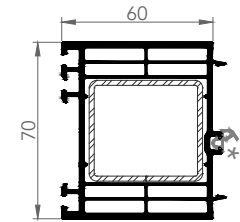
7281 70x60 mm YÜKSELTME
