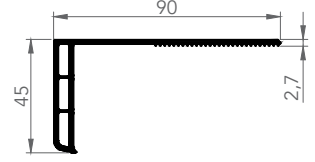
6055 İNCE TIRTIKLI PERVAZ
