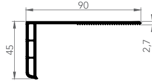
6055 İNCE TIRTIKLI PERVAZ
