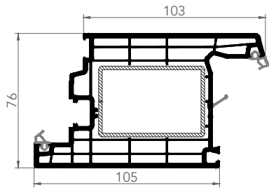
7646E KAPI KANAT
