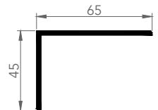
6056 L-PERVAZ
