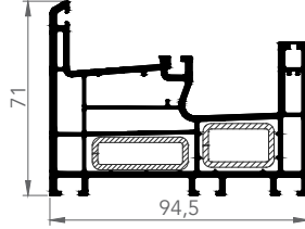
SÜRME SABİT KASA
