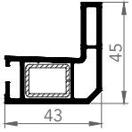
7407 SİNEKLİK RAY
