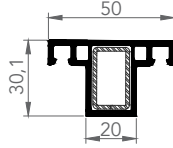
7409 SİNEKLİK KANAT İÇİ ORTA KAYIT
