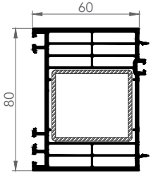
7283 80x60 mm YÜKSELTME
