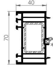
7280 70x40 mm YÜKSELTME
