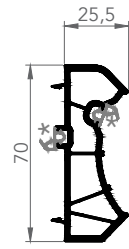
7255 KÖŞE DÖNÜŞ ADAPTÖRÜ
