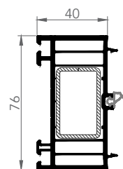
7665 76/40 YÜKSELTME
