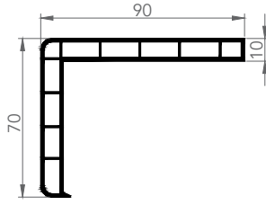
6019 KALIN PERSİYAN
