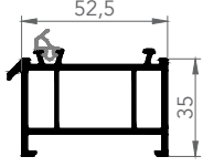
7666 KÖR KASA YÜKSELTME
