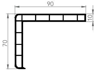
6019 KALIN PERVAZ
