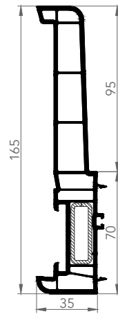
DENİZLİK FRANSA
