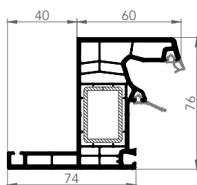
7607E PERVAZLI KASA
