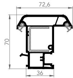
HAREKETLİ ORTA KAYIT
