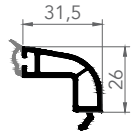
7652 ÇİFT CAM ÇİTASI 24 mm
