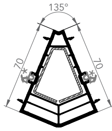
7253 KÖŞE DÖNÜŞ "135 DERECE"
