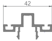
AB01014 ALIN ALINA BAĞLANTI-6661
