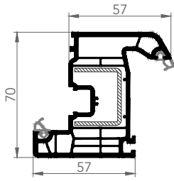
KANAT
