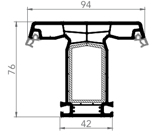
7636AE ORTA KAYIT
