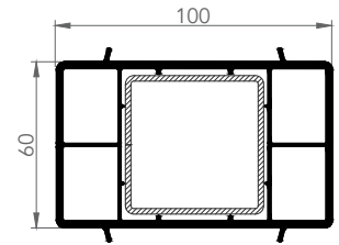
6051 60x100 ODACIKLI KUTU PROFİLİ
