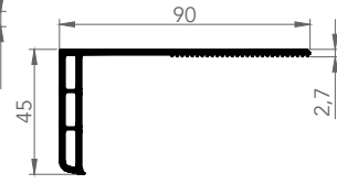
6055 İNCE TIRTIKLı PERSİYAN
