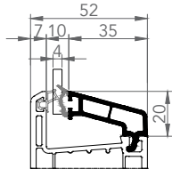
6306 TEK CAM ÇİTASI 4mm
