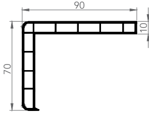
6019 KALIN PERVAZ
