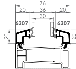
6307-6307 ÇİFT CAM ÇİTASI 30mm
