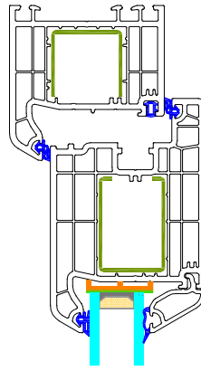
BB - DETAYI
