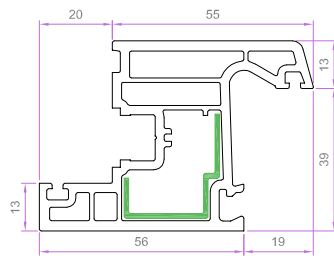
KANAT PROFİLİ 5202 1.192 kg/m 5202 EU-B 1.049 kg/m
