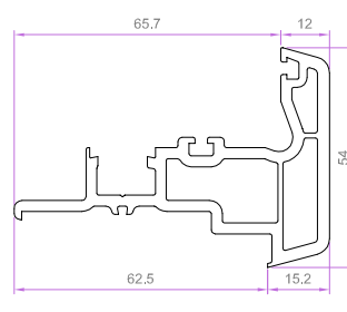
HAREKETLİ ORTA KAYIT PROFİLİ 6006 0.985 kg/m
