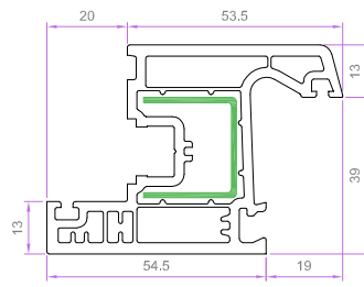
YENİ KANAT PROFİLİ 5212 1.170 kg/m 5212 EU-B 1.059 kg/m
