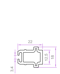
KANAT DOLGU ALIN PR. 7410 0.197 kg/m
