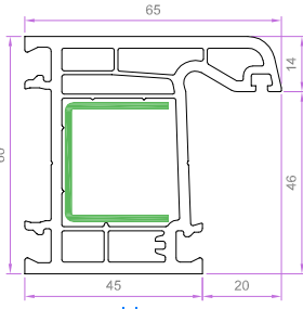
KASA PROFİLİ 6041 1.243 kg/m 6041 EU-B 1.032 kg/m
