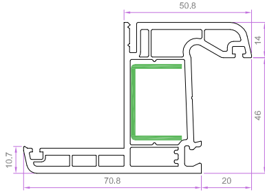
PERVAZLI KASA PROFİLİ 6054 1.295 kg/m
