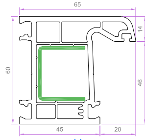
KASA PROFİLİ 6031 1.210 kg/m 6031 EU-B 1.004 kg/m
