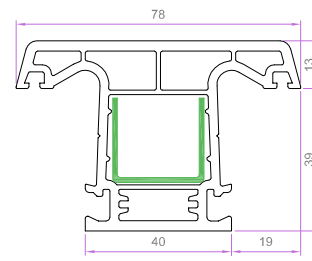
ORTA KAYIT PRF. 5203 1.197 kg/m 5203 EU-B 1.076 kg/m
