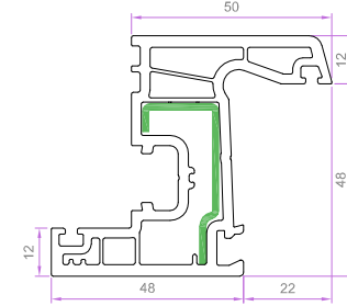
HAYAT EKONOMİK KANAT 6240 1.199 kg/m 6236 EU-B 1.055 kg/m
