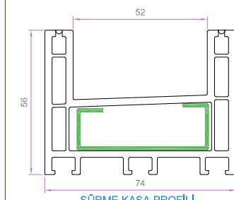
SÜRME KASA PROFİLİ 7401 1.373 kg/m
