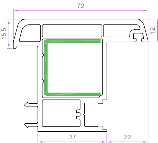
HAREKETLİ O.KAYIT PROFİLİ 6029 1.117 kg/m
