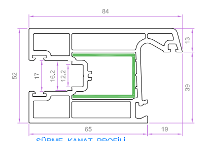
SÜRME KANAT PROFİLİ 7402 1.468 kg/m
