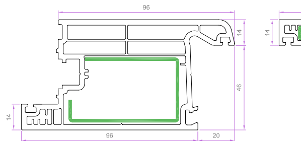
KAPI KANAT PROFİLİ 'İÇERİ AÇILAN' 6045 1.834 kg/m
