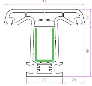
DAR ORTA KAYIT PRF. 6143 1.194 kg/m 6143 EU-B 1.051 kg/m
