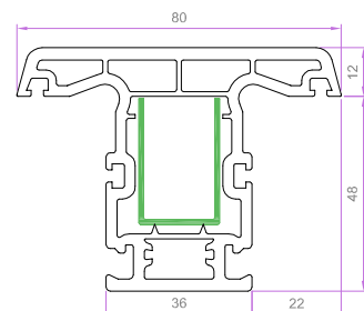
ORTA KAYIT PROFİLİ 6005 1.391 kg/m
