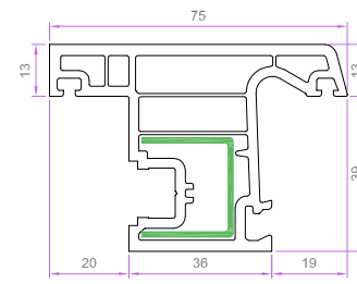
DIŞARI AÇILAN PENCERE KANAT 5209 1.177 kg/m
