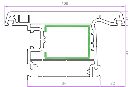
HAYAT KAPI KANAT PRF. (DIŞARI AÇILAN) 6242 1.695 kg/m 6238 EU-B 1.517 kg/m
