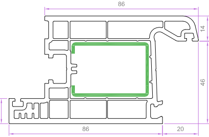
YENİ KAPI KANAT PRF. (İÇERİ AÇILAN) 6145 1.728 kg/m 6145 EU-B 1.511 kg/m
