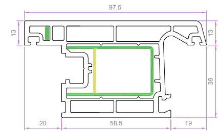
DIŞARI AÇILAN KAPI KANAT PROFİLİ 5210 1.502 kg/m
