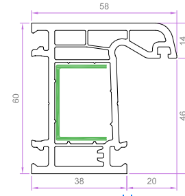
DAR KASA PROFİLİ 6141 1.099 kg/m 6141 EU-B 0.974 kg/m
