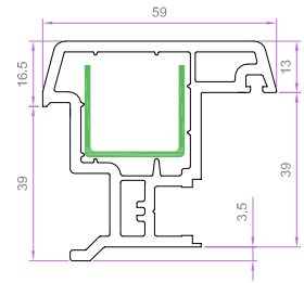
H. ORTA KAYIT PROFİLİ 5207 0.940 kg/m
