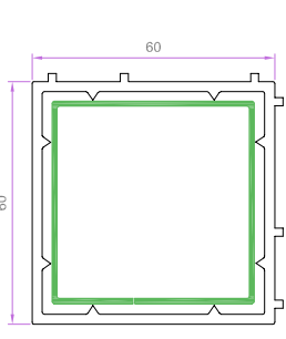
60x60 KUTU PROFİLİ 6020 0.905 kg/m
