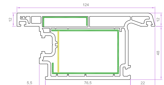
KAPI KANAT PROFİLİ 'DIŞARI AÇILAN' 6008 1.834 kg/m
