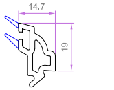
ÇİFTCAM ÇİTASI 5206 0.208 kg/m
