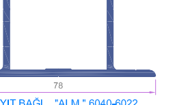
O.KAYIT BAĞL. "ALM." 6040-6022 3101 1.001 kg/m
