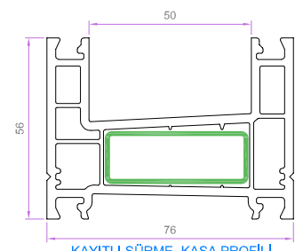
KAYITLI SÜRME KASA PROFİLİ 7406 1.361 kg/m
