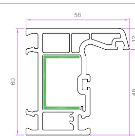
EKO KASA PROFİLİ 6001 1.136 kg/m
