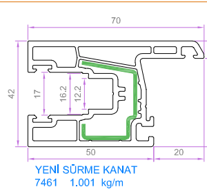
YENİ KAYITLI SÜRME KASA 7460 1.068 kg/m
