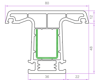
HAYAT EKO O.KAYIT PRF. 6233 1.215 kg/m 6235 EU-B 1.107 kg/m
