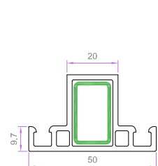
SİNEKLİK KANAT İÇİ KAYIT 7409 0.459 kg/m
