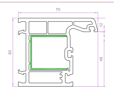
SÜPER KASA PROFİLİ 6002 1.304 kg/m
