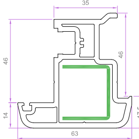
HAREKETLİ ORTA KAYIT PROFİLİ 6044 1.078 kg/m
