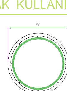
ADAPTÖR BORUSU 6016 0.621 kg/m
