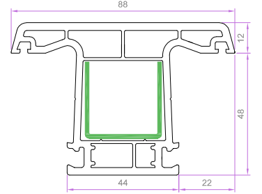
HAYAT ORTA KAYIT PROFİLİ 6023 1.411 kg/m 6025 EU-B 1.281 kg/m
