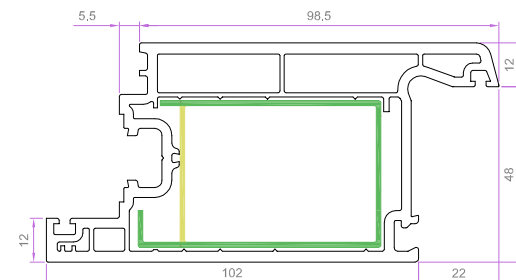
KAPI KANAT PROFİLİ 'İÇERİ AÇILAN' 6007 1.821 kg/m
