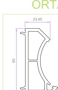
KÖŞE DÖNÜŞ ADAPTÖRÜ 6015 0.678 kg/m
