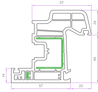
KANAT PROFİLİ (5-ODACIKLI) 7152 1.458 kg/m 7152 EU-B 1.300 kg/m
