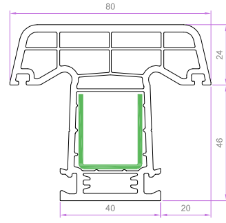
ORTA KAYIT PRF. (5-ODACIKLI) 7153 1.491 kg/m 7153 EU-B 1341 kg/m
