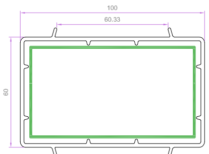
60x100 ODACIKSIZ KUTU PROFİLİ 6052 0.986 kg/m
