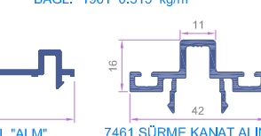
7461 SÜRME KANAT ALIN BAĞL. 6661 0.465 kg/m
