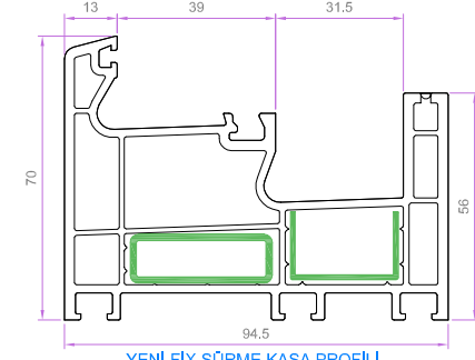
YENİ FIX SÜRME KASA PROFİLİ 7411 1.625 kg/m
