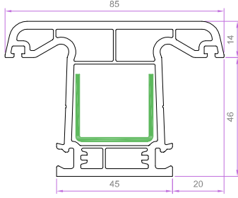
ORTA KAYIT PROFİLİ 6033 1.396 kg/m 6033 EU-B 1.236 kg/m
