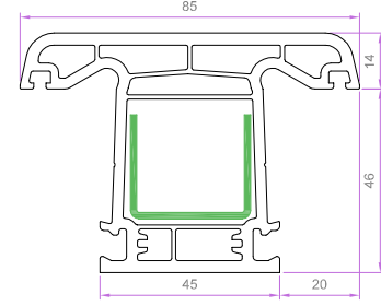
ORTA KAYIT PROFİLİ 6043 1.433 kg/m 6043 EU-B 1.187 kg/m
