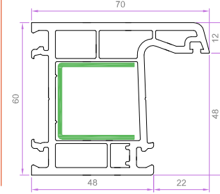
HAYAT KASA PROFİLİ 6022 1.279 kg/m 6024 EU-B 1.167 kg/m
