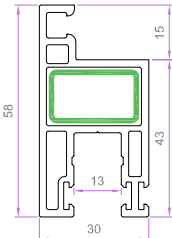
SİNEKLİK SÜRME KANAT 7408 0.644 kg/m
