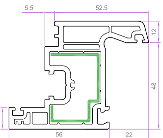
NORMAL KANAT PROFİLİ 6003 1.330 kg/m
