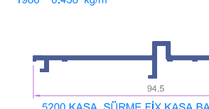
5200 KASA, SÜRME FIX KASA BAĞL. "ALM." 2485 0.560 kg/m
