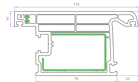
KAPI KANAT PROFİLİ 'DIŞARI AÇILAN' 6048 1.832 kg/m
