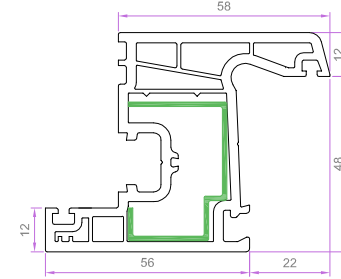
HAYAT KANAT PROFİLİ 6027 1.332 kg/m 6028 EU-B 1.232 kg/m
