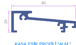
KASA EŞİK PROFİLİ "ALM." 3308 0.668 kg/m
