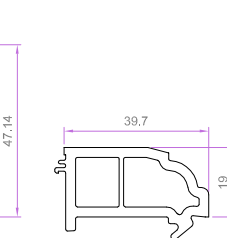
SÜRME FIX KASA KAPAMA 7405 0.468 kg/m
