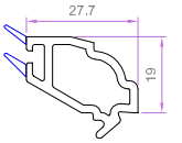
TEKCAM ÇİTASI 5205 0.281 kg/m
