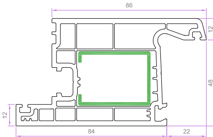
HAYAT KAPI KANAT PRF. (İÇERİ AÇILAN) 6241 1.892 kg/m 6237 EU-B 1.511 kg/m
