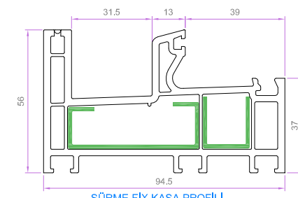
SÜRME FIX KASA PROFİLİ 7403 1.595 kg/m
