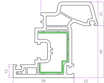
DAMLALIKLI KANAT PROFİLİ 6004 1.434 kg/m
