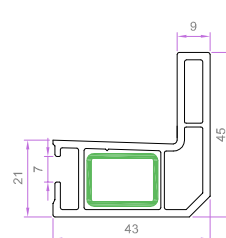
SİNEKLİK RAY KASA 7407 0.520 kg/m
