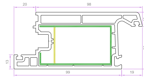
KAPI KANAT PROFİLİ 5204 1.616 kg/m
