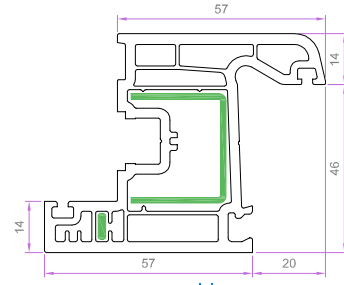
KANAT PROFİLİ 6042 1.403 kg/m 6042 EU-B 1.156 kg/m
