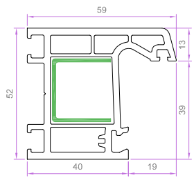
KASA PROFİLİ 5201 1.018 kg/m 5201 EU-B 0.901 kg/m
