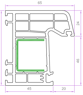
KASA PRF. (5-ODACIKLI) 7151 1.382 kg/m 7151 EU-B 1.245 kg/m
