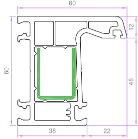
HAYAT EKO KASA 6232 1.062 kg/m 6234 EU-B 0.965 kg/m
