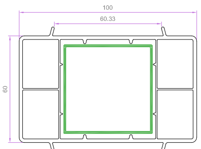
60x100 ODACIKLI KUTU PROFİLİ 6051 1.148 kg/m
