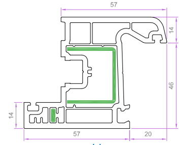
KANAT PROFİLİ 6032 1.374 kg/m 6032 EU-B 1.224 kg/m
