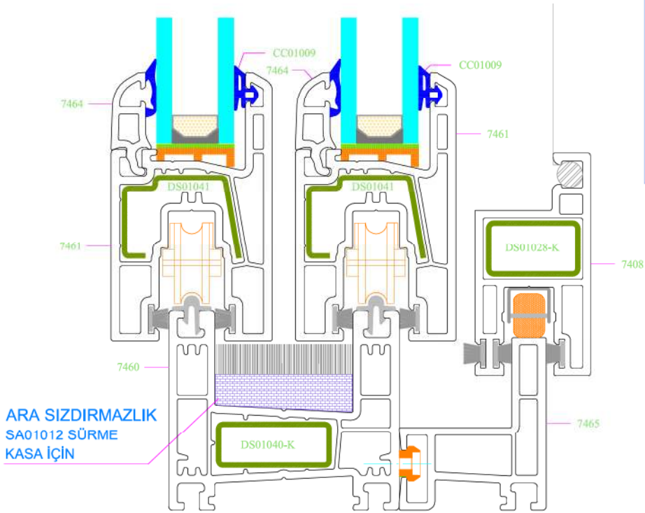
KANAT BİRLEŞİM DETAYLARINDA SU VE RÜZGAR GEÇİŞİNİ ENGELLEMELİK İÇİN KULLANILAN SIZDIRMAZLIK AKSESUARİ
